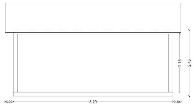
ELEVACIÓN LATERAL 1 (DORMITORIOS)
