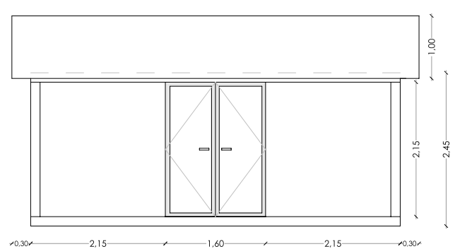
ELEVACIÓN LATERAL 2 (LIVING - COCINA)
