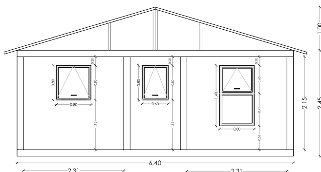
ELEVACIÓN POSTERIOR
